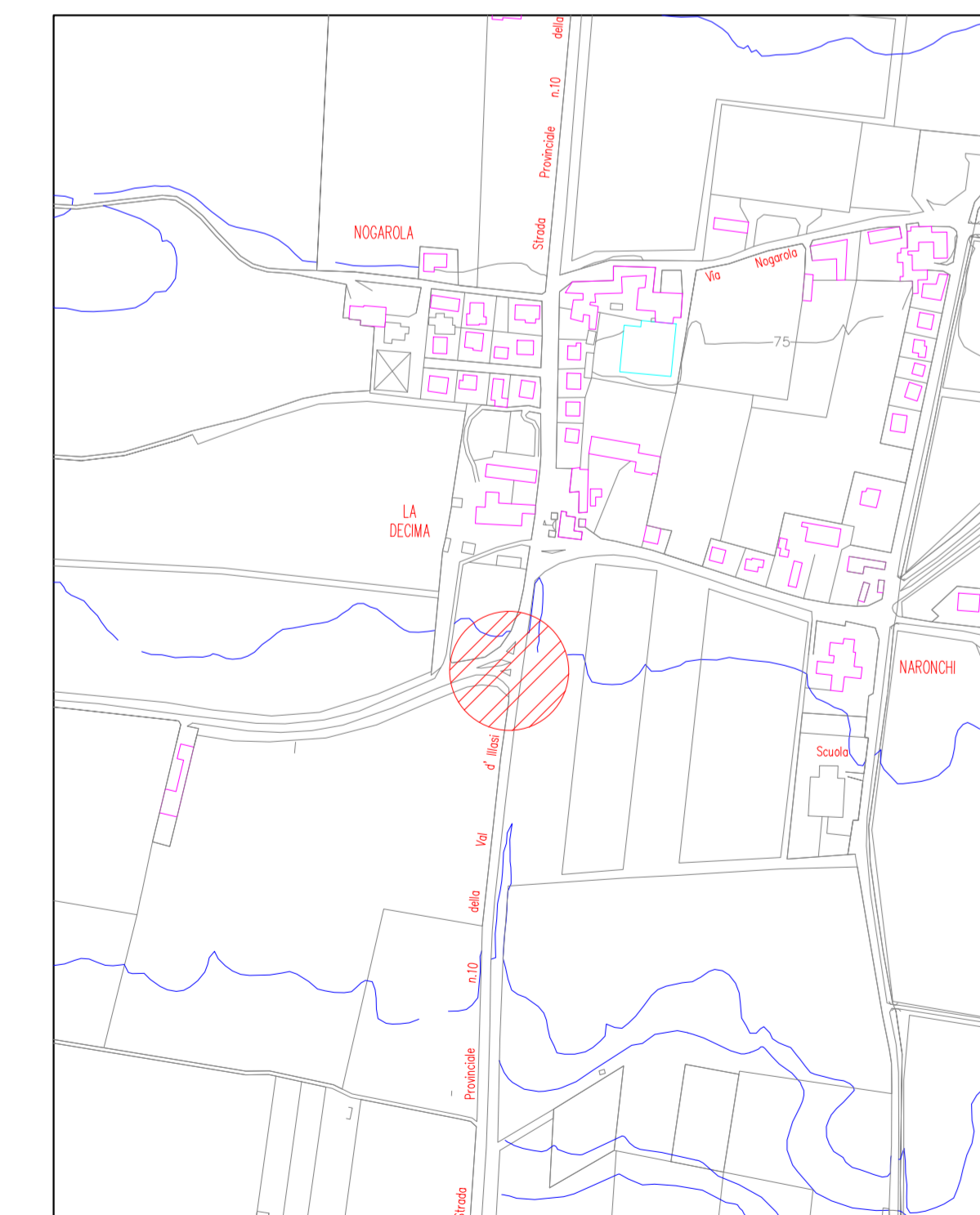
STRALCIO CATASTALE - SCALA 1:5.000
